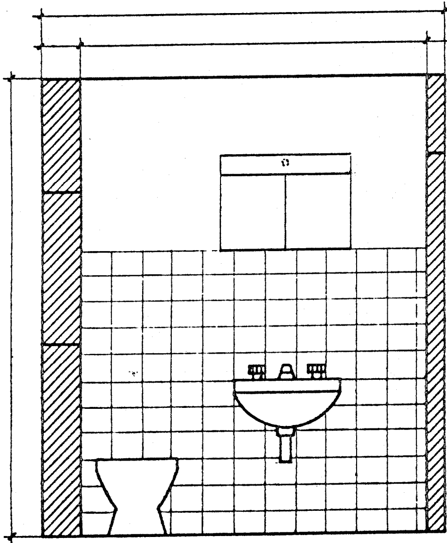
COUPE : F
